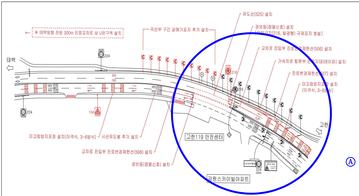
[그림 2] 미끄럼방지포장 설치 기준 미이행 사례
